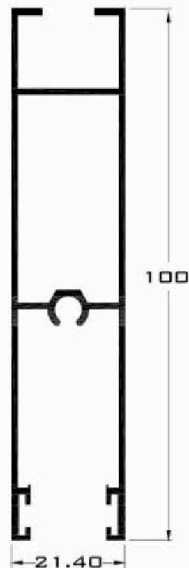
3559 ZOCALO DOBLE VIDRIO
