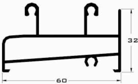
3501 CERCO INFERIOR
