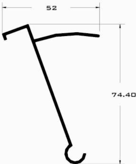
3518 ESQUINERO REGULABLE HEMBRA
