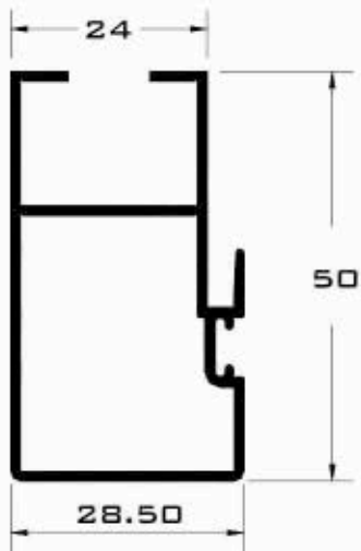
3504 HOJA CENTRAL
