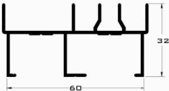
3508 CERCO LATERAL
