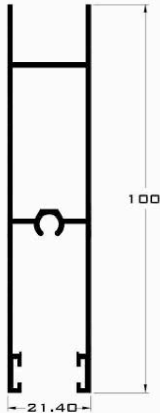
3560 ZOCALO
