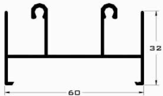
3502 CERCO SUPERIOR
