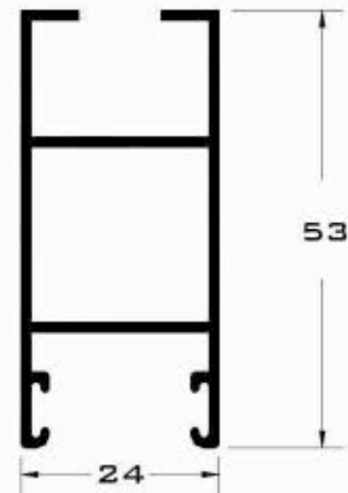
3505 HOJA LATERAL
